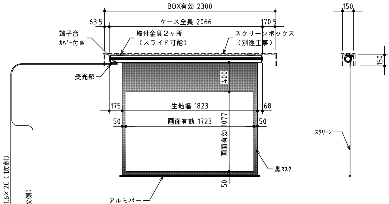
外観図 1/30
