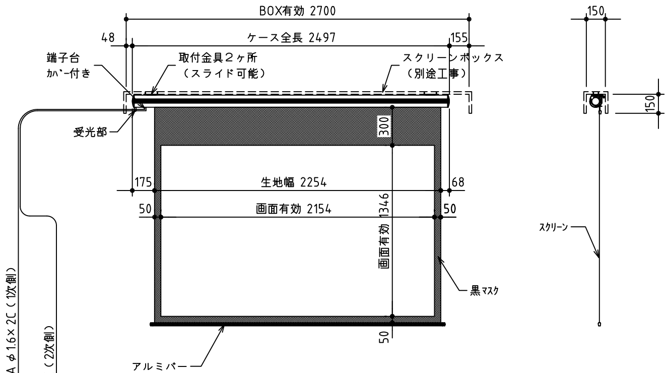
外観図 1/30
