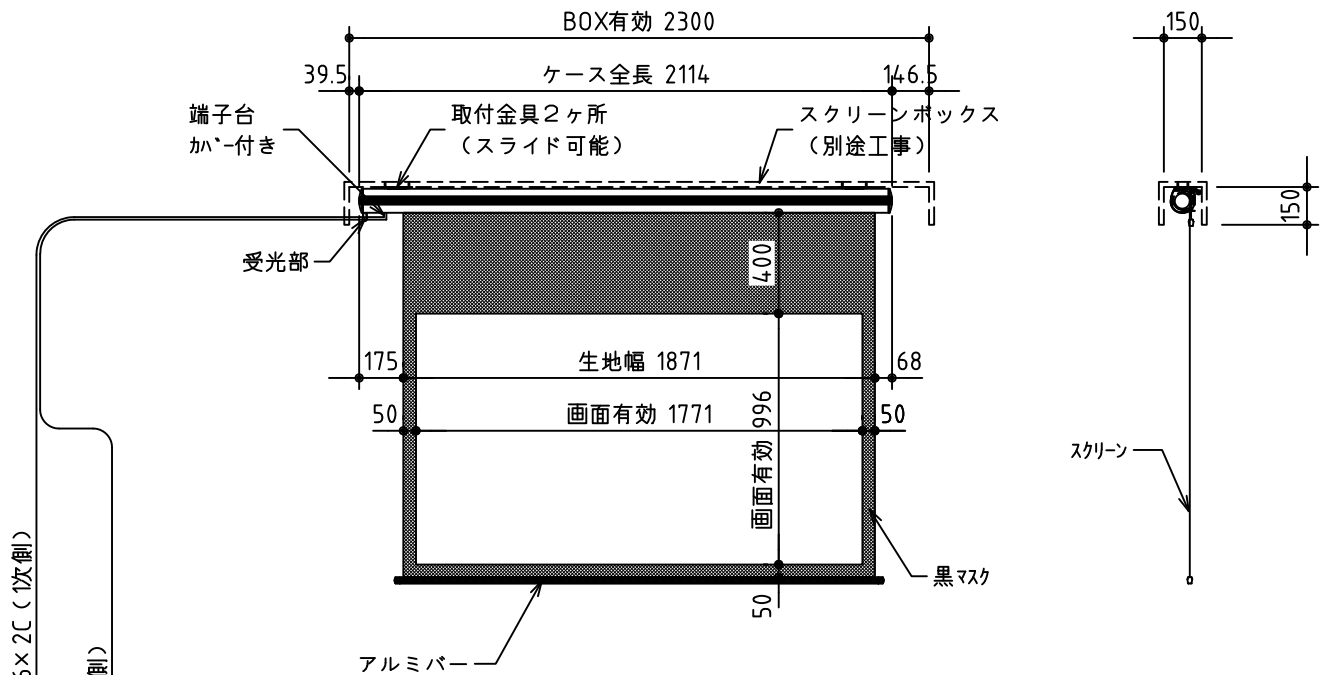
外観図 1/30
