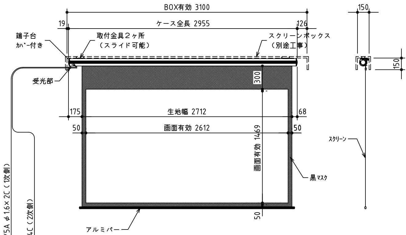
外観図 1/30
