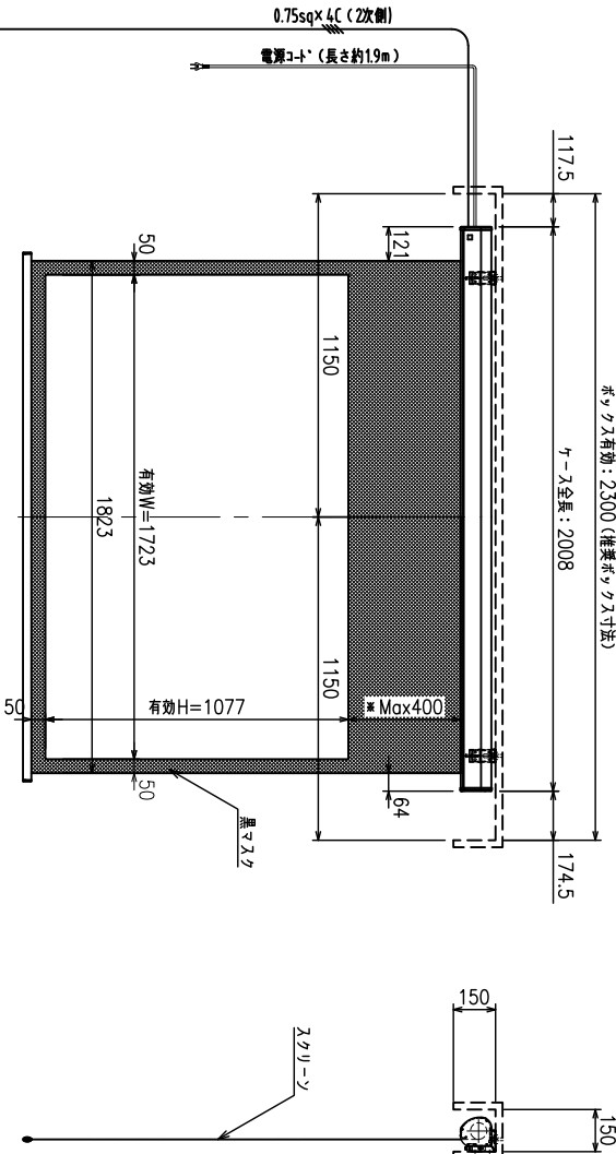
外観図 S=1/20
