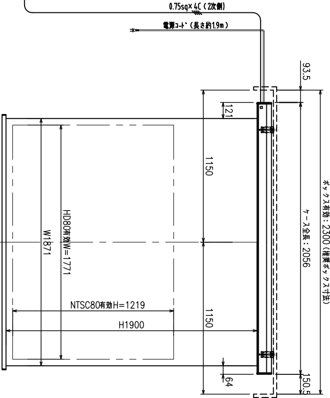
外觀図 S=1/20
