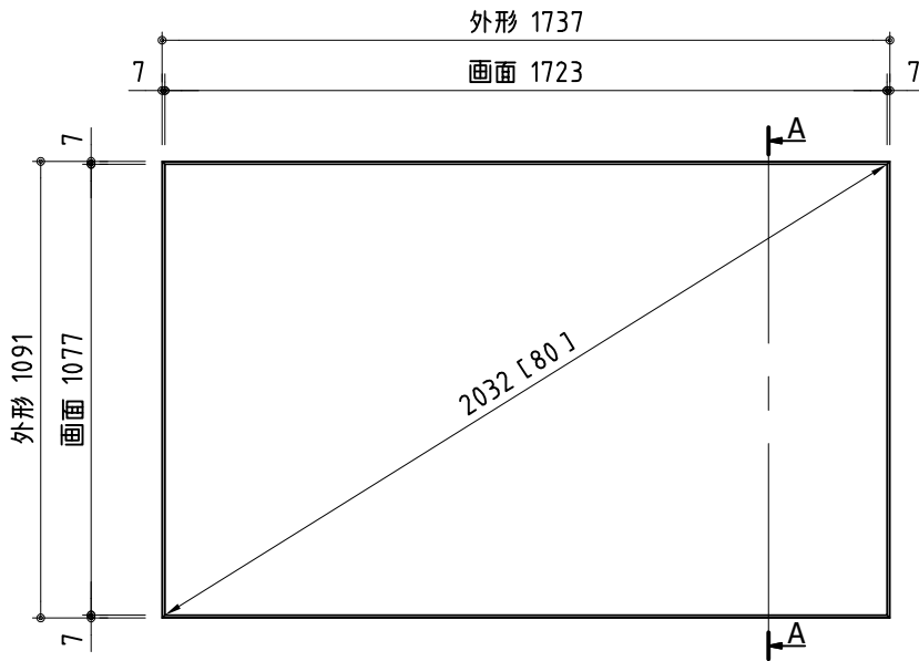
外観図(正面) S=1/20
