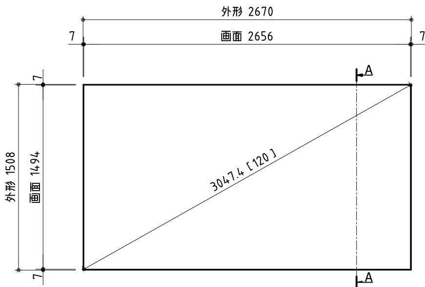
外観図(正面) S=1/30
