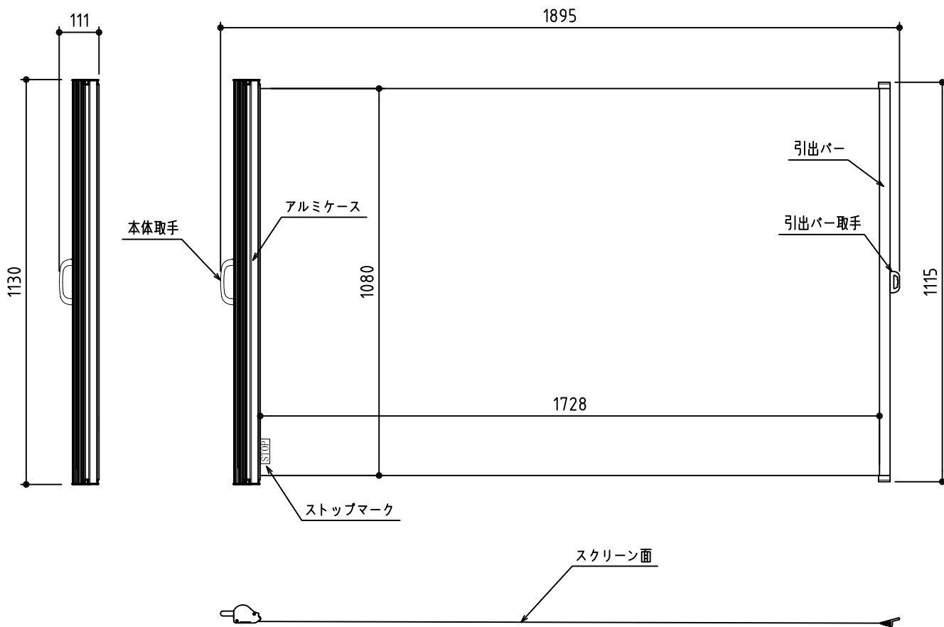
外觀図 S=1/15
