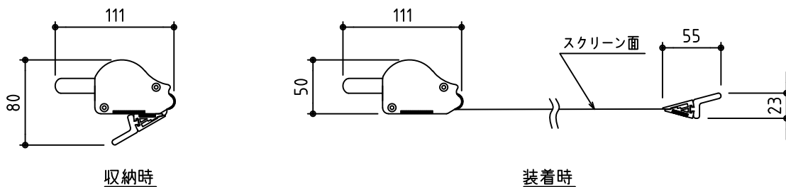
詳細図 S=1/5
