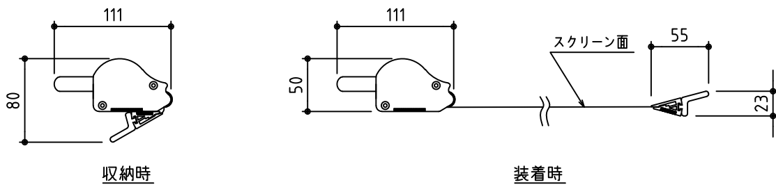
詳細図 S=1/5
