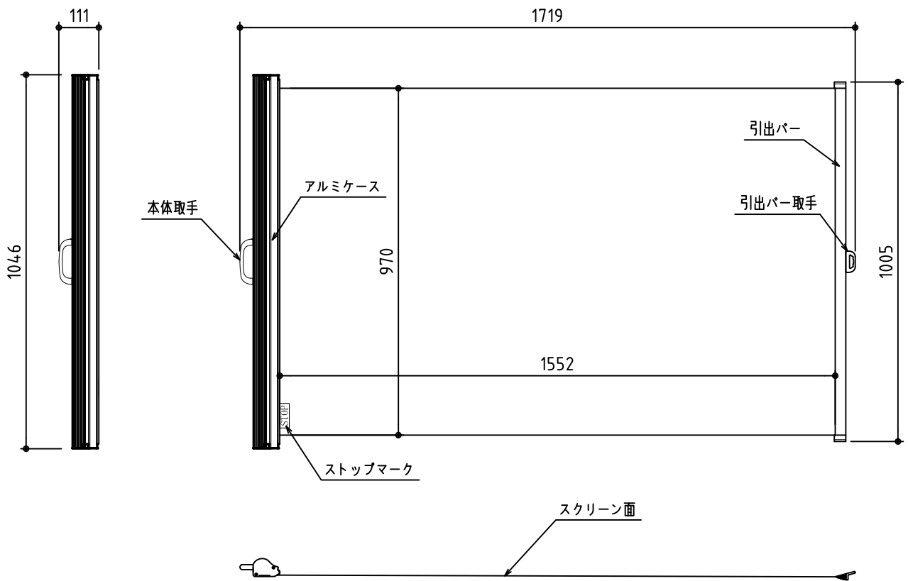
外觀図 S=1/15
