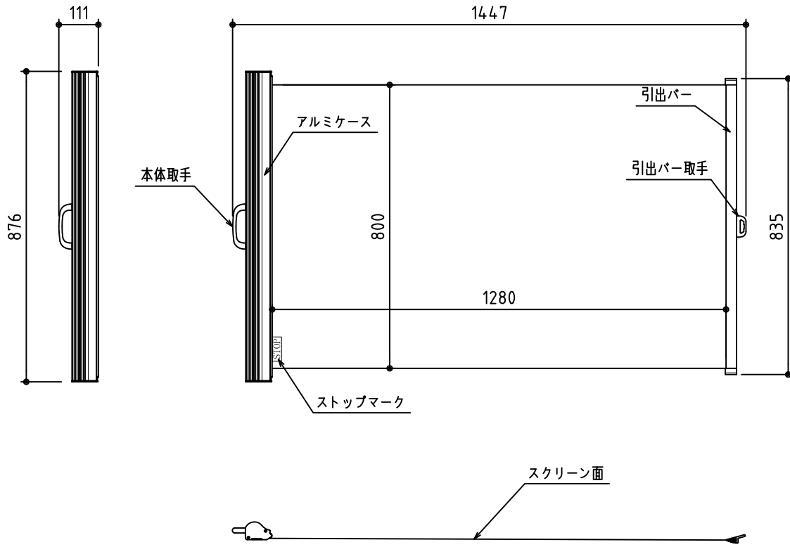
外觀図 S=1/15
