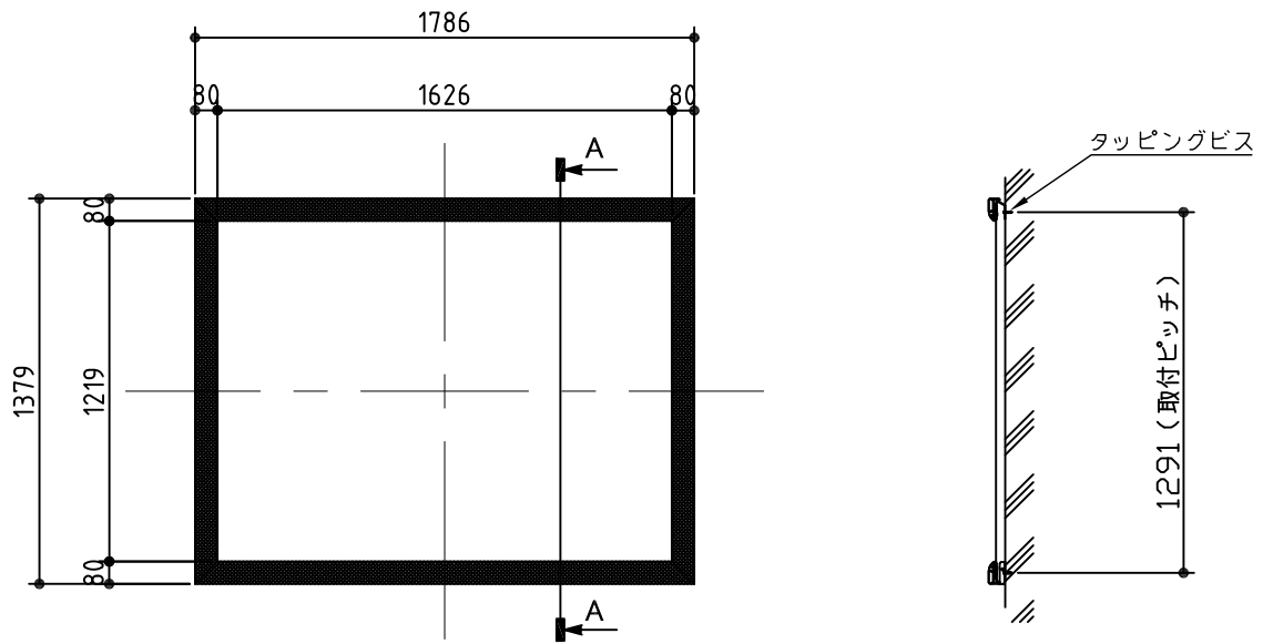
外観図 S=1/30
