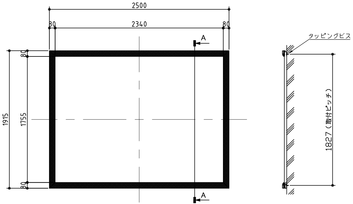
外観図 S=1/30
