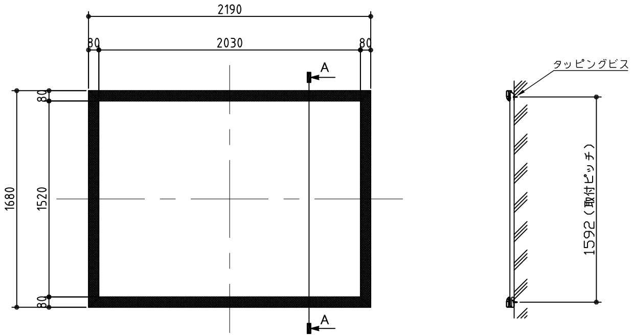
外観図 S=1/30
