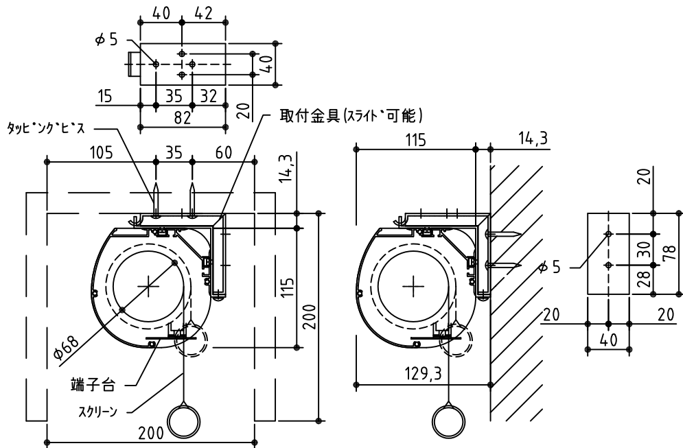
ホックス取付時 S=1/5
