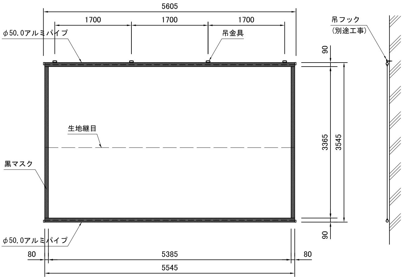
外観図 S=1/50
