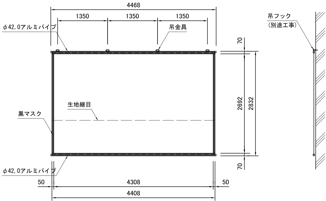
外観図 S=1/50
