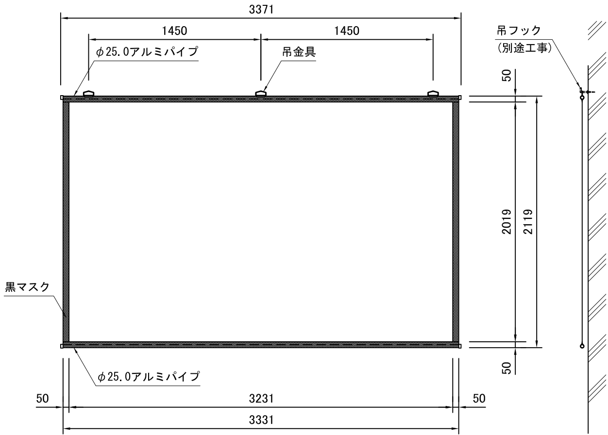
外観図 S=1/30
