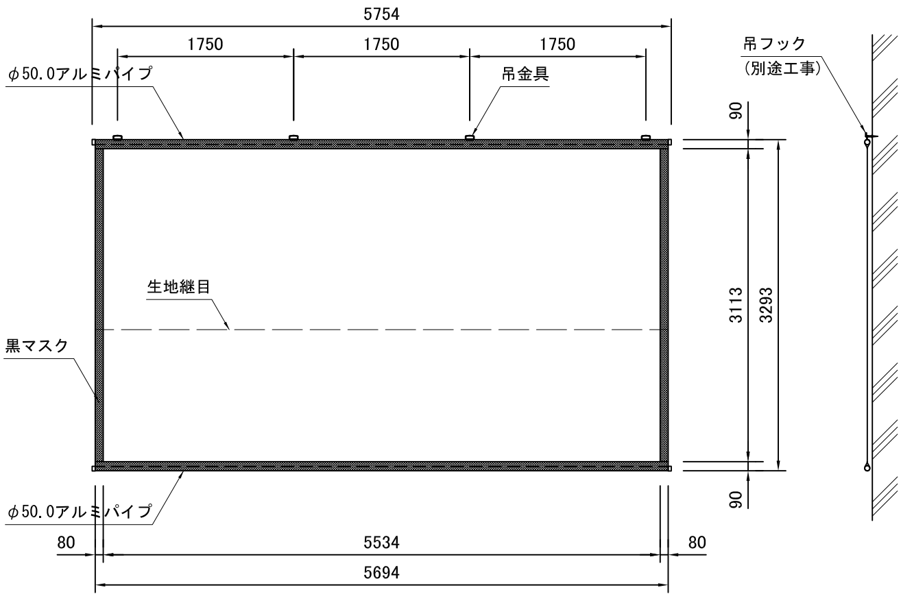
外観図 S=1/50
