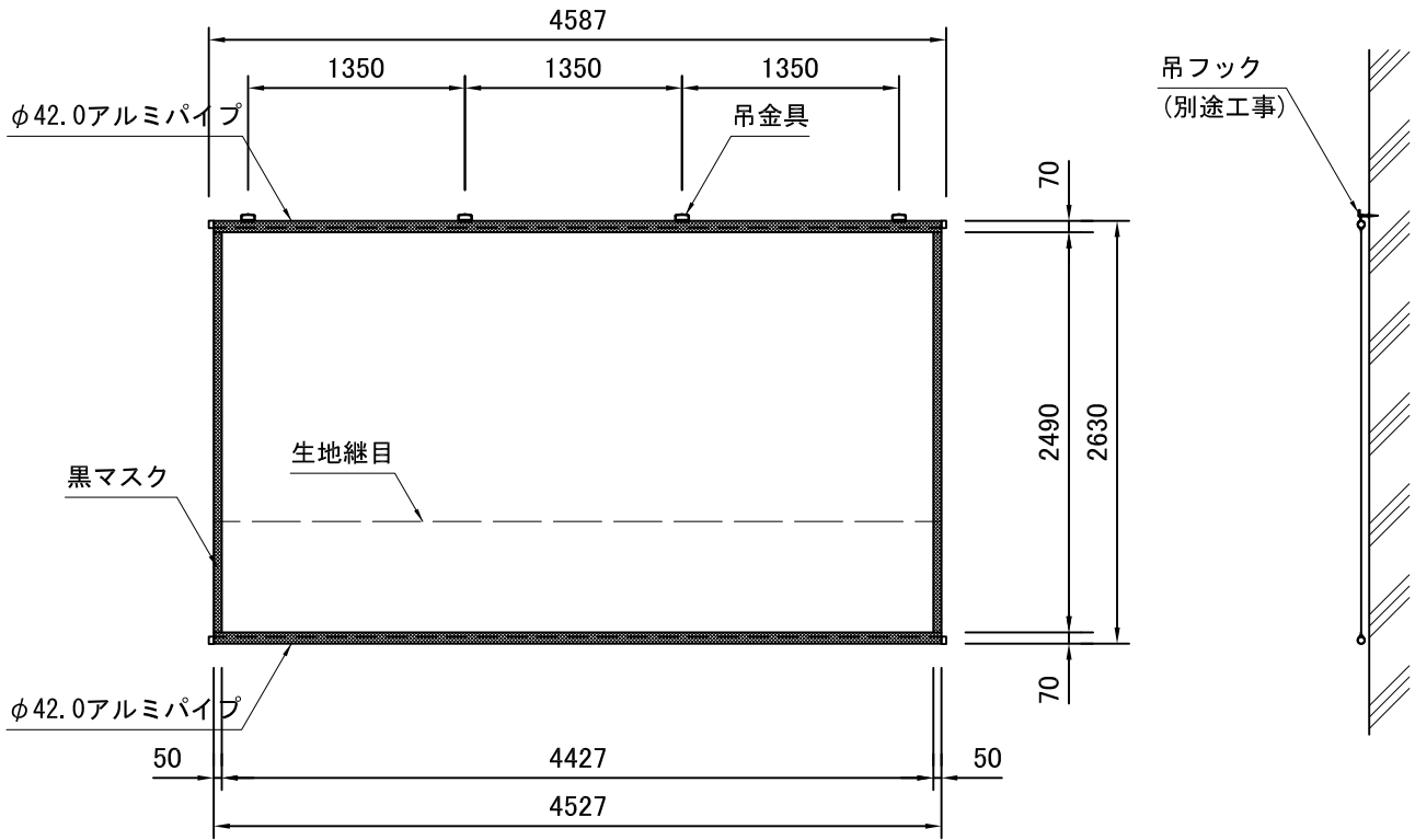
外観図 S=1/50
