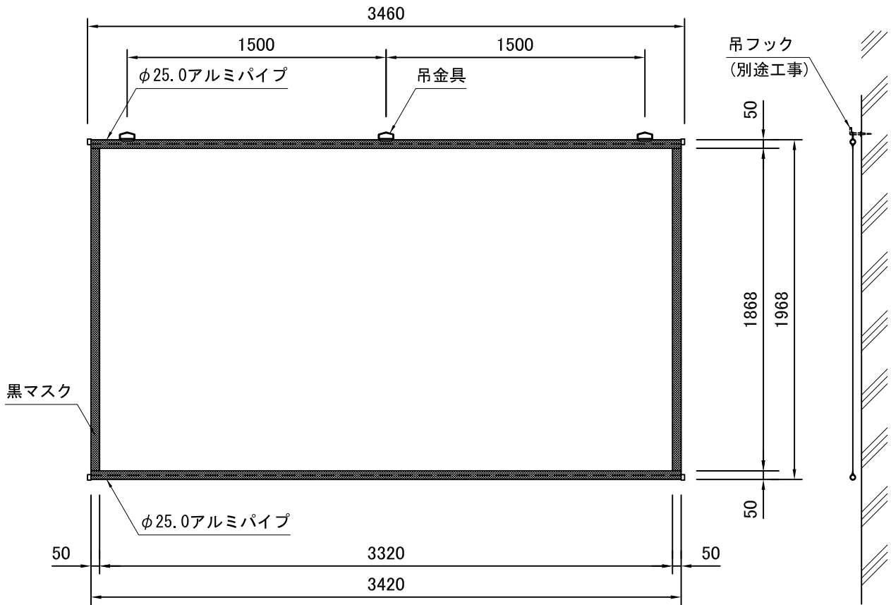
外觀図 S=1/30
