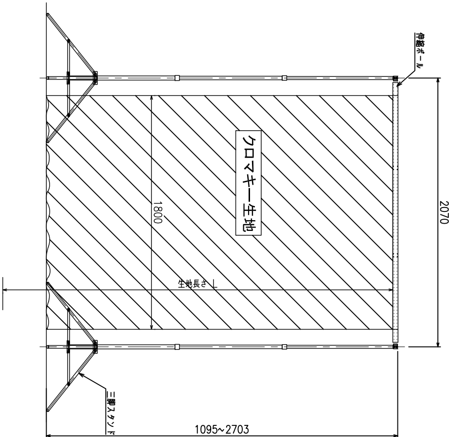
正面図
