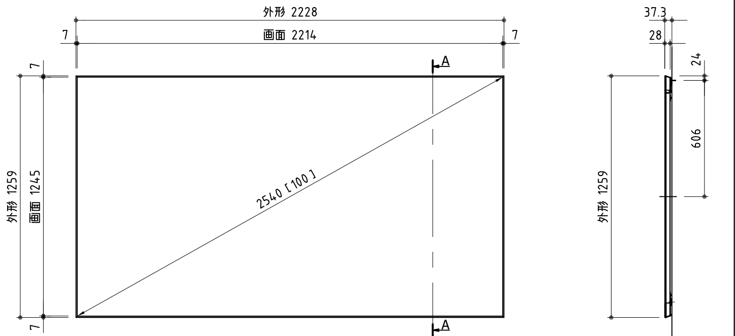
外観図(正面) S=1/20
