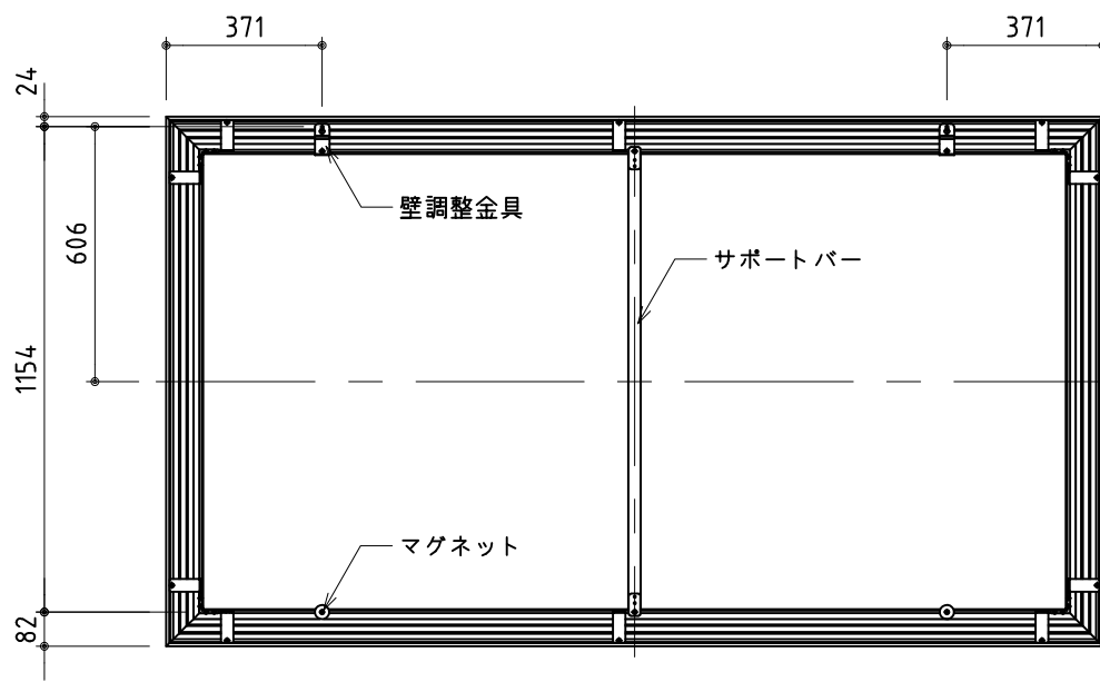
外観図(背面) S=1/20
