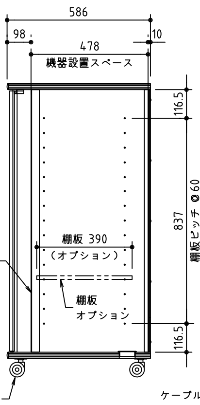
断面
