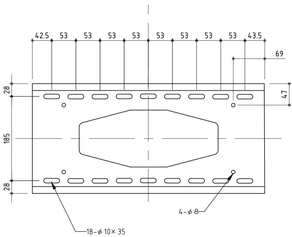
壁側金具
