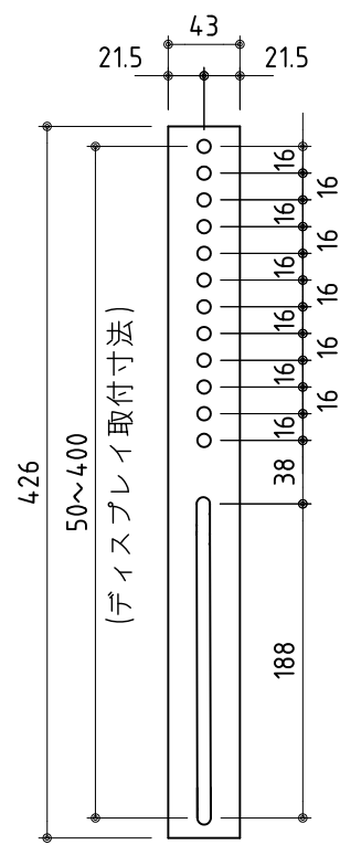
TV側金具
