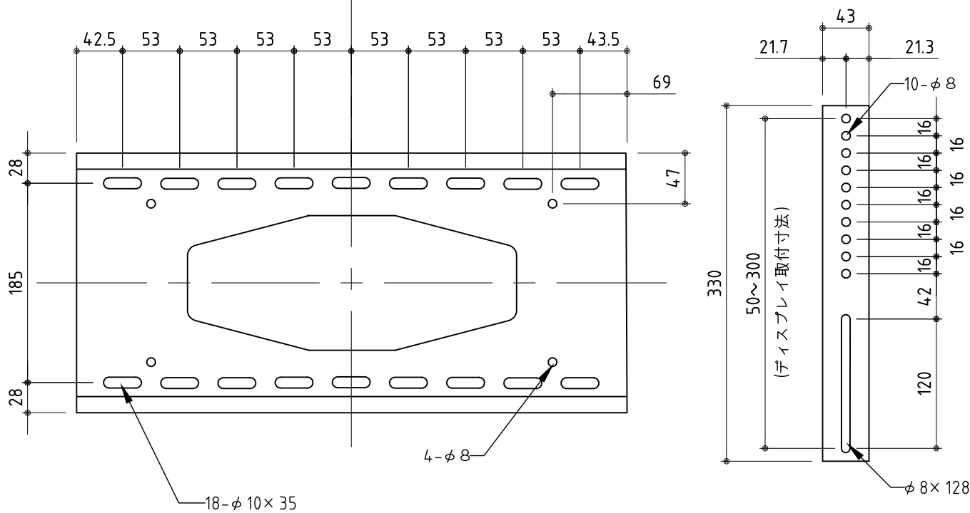
TV側金具
