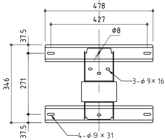
ベースプレート (プラスチックカバー外した状態)
