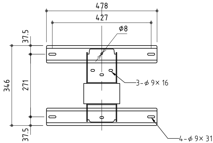
ベースプレート (プラスチックカバー外した状態)
