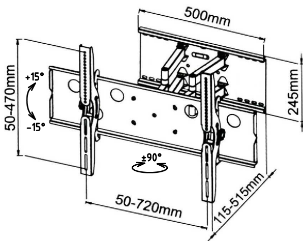
壁側ウォールプレート
