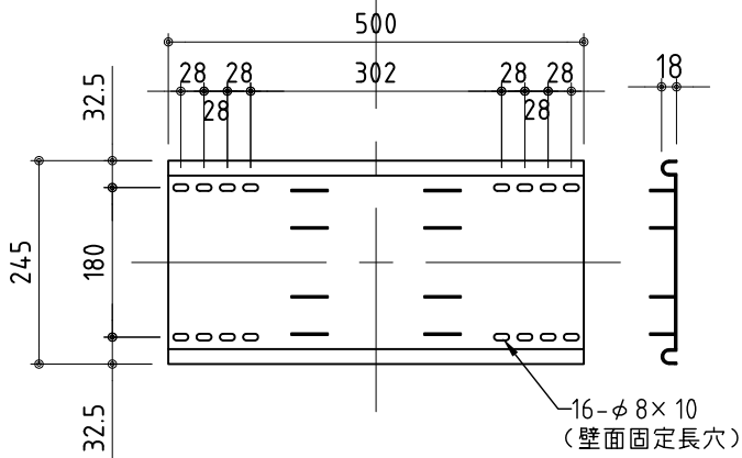
壁側ウォールプレート
