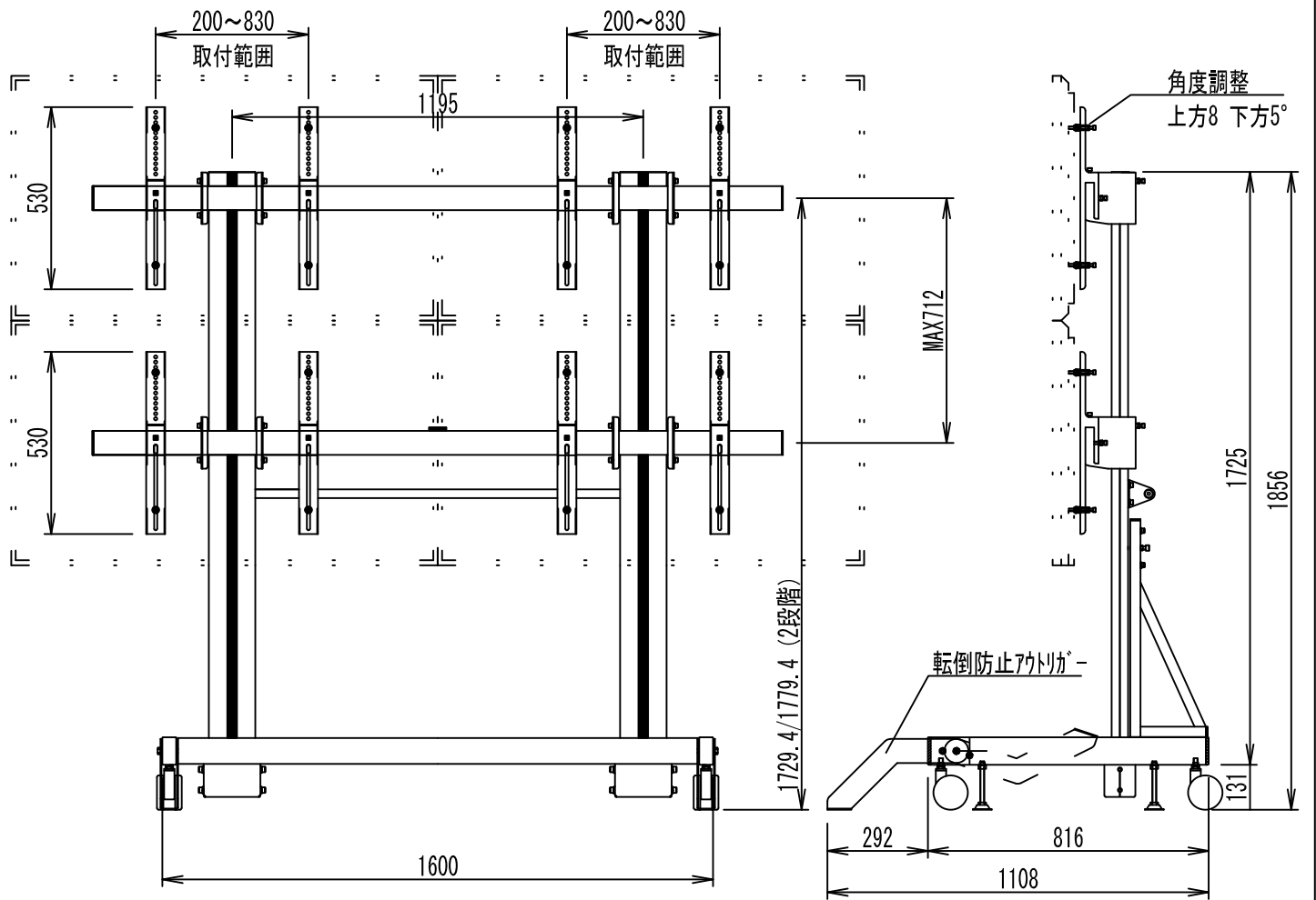
アタッチメント穴位置図 S=1/10
